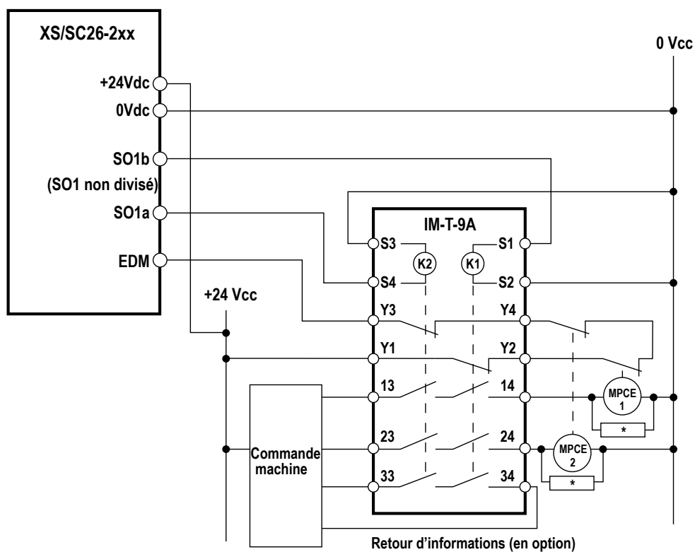
Illustration 44. Raccordement générique du XS/SC26-2 : sortie de sécurité électronique à l'IM-T-9A
