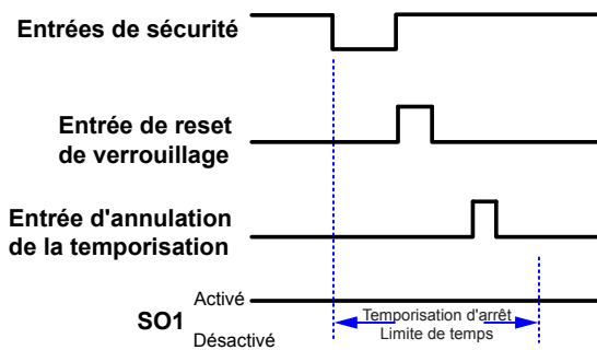
Illustration 29. Fonction Maintien de la sortie activée pour les entrées de sécurité avec reset de verrouillage
