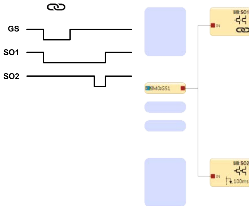
Illustration 34. Chronogramme — Sorties de sécurité liées
