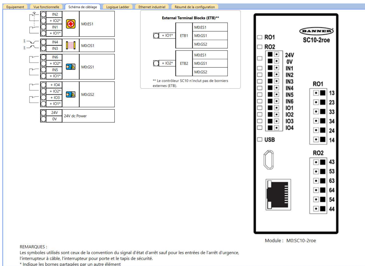
Illustration 247. Onglet Schéma de câblage avec trois boutons d'arrêt d'urgence et des borniers externes
