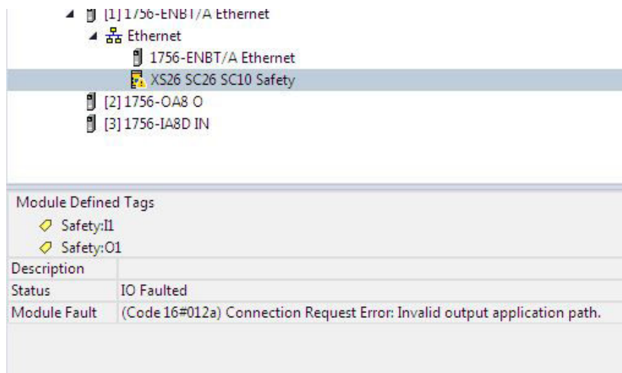
Illustration 163. Incorrect : utilisation de la connexion « État/Défaut VI » sur un contrôleur de sécurité qui ne prend pas en charge cette fonction.
