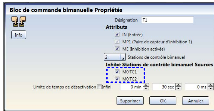
Illustration 145. Options d'inhibition de commande bimanuelle
