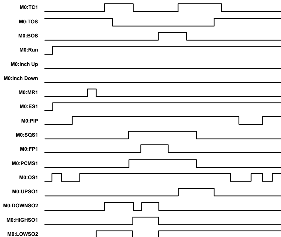
Illustration 139. Commande presse — Diagramme temporel, paramétrage manuel Course montante
