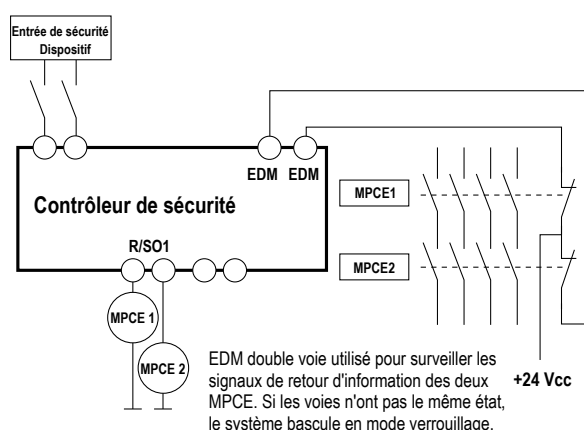
Illustration 38. Raccordement de l'EDM à deux canaux
