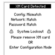
Illustration 270. Modèles XS/SC26-2de : verrouillage du système
