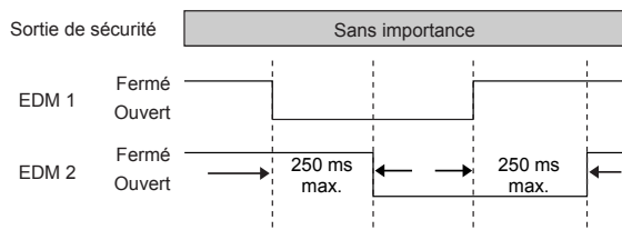
Illustration 40. Logique de temporisation : EDM à deux canaux, temporisation entre les canaux
