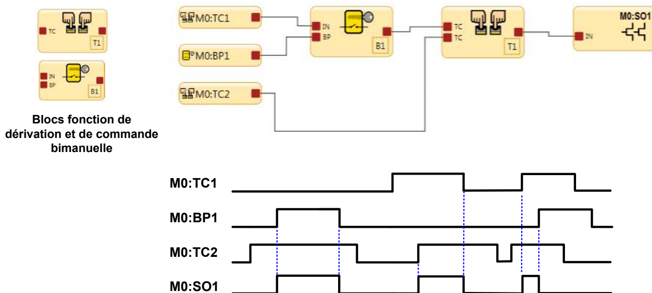
Illustration 144. Chronogramme — Bloc de commande bimanuelle et blocs de dérivation avec 2 entrées de commande bimanuelle
