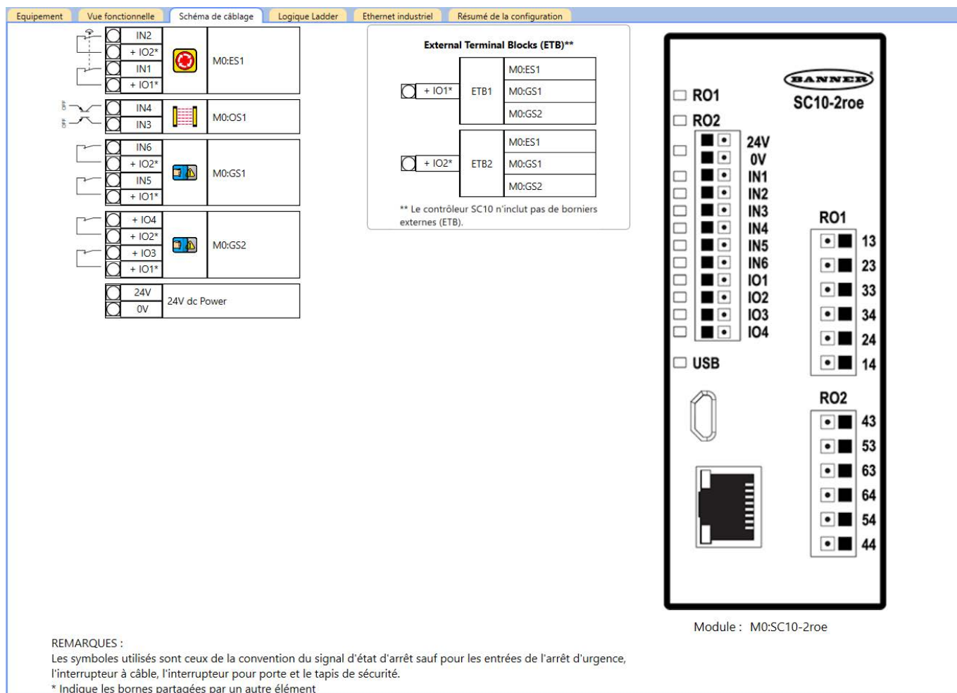
Illustration 77. Onglet Schéma de câblage — SC10-2 avec borniers externes
