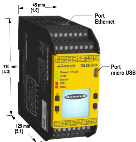
Illustration 10. Dimensions du module de base XS/SC26-2
