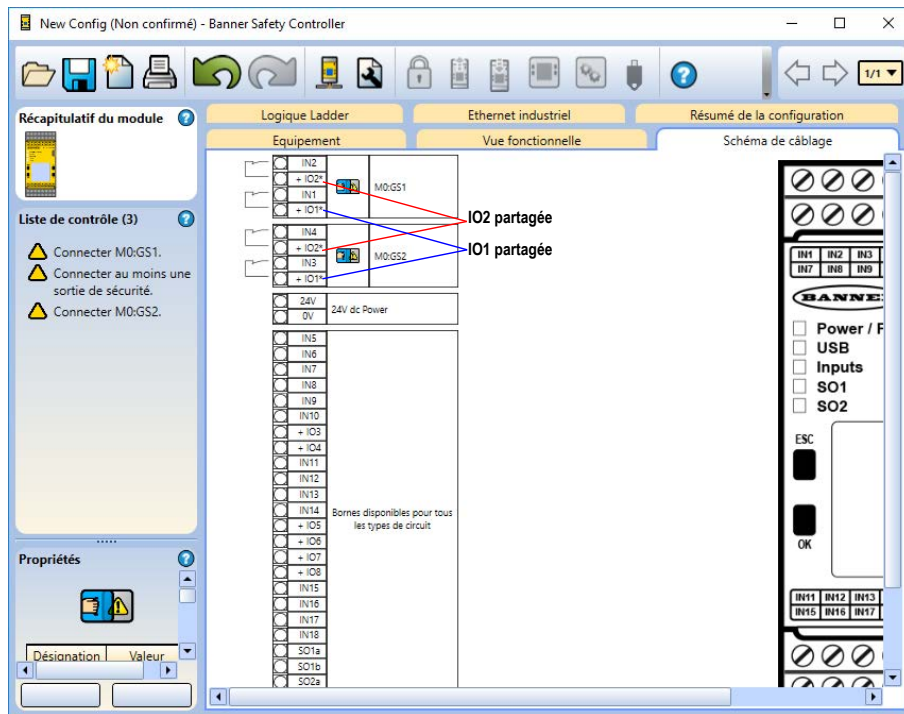
Illustration 5. Onglet Schéma de câblage avec les E/S partagées
