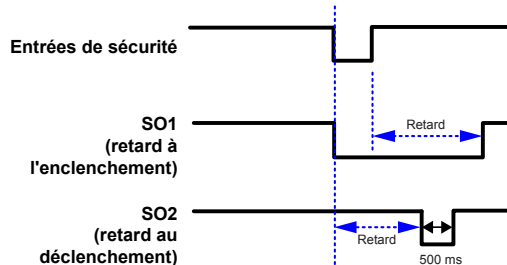
Illustration 31. Chronogramme — Retards à l'enclenchement et au déclenchement généraux d'une sortie de sécurité
