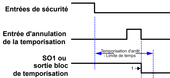
Illustration 20. L'entrée de sécurité reste en mode d'arrêt.
