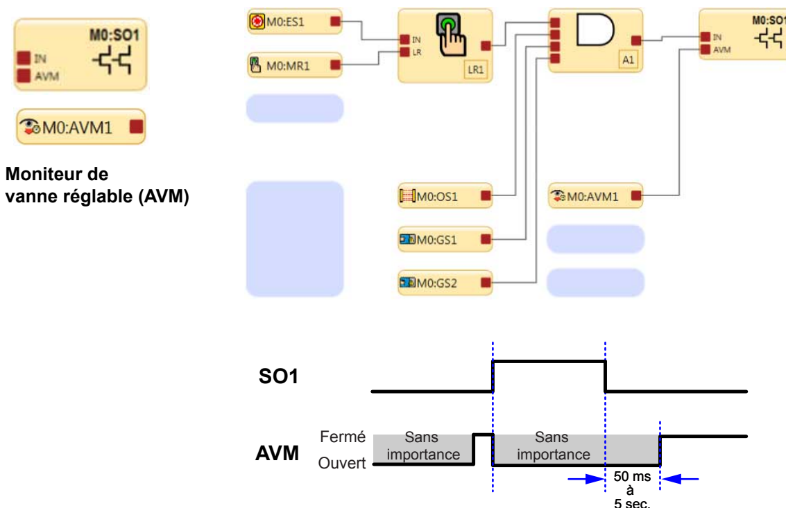
Illustration 19. Logique de temporisation — Fonction AVM
