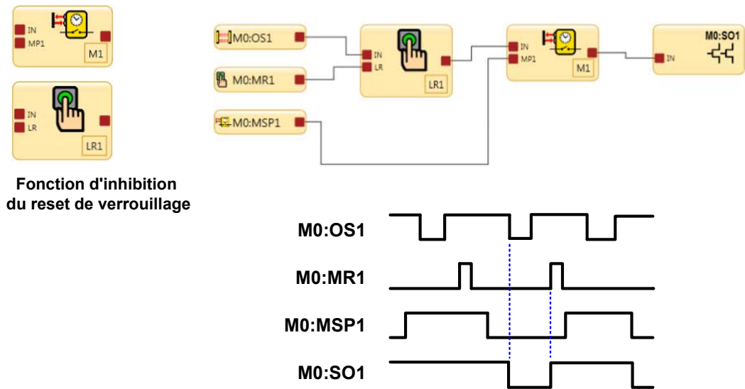
Illustration 117. Chronogramme — Bloc de reset à verrouillage et bloc d'inhibition
