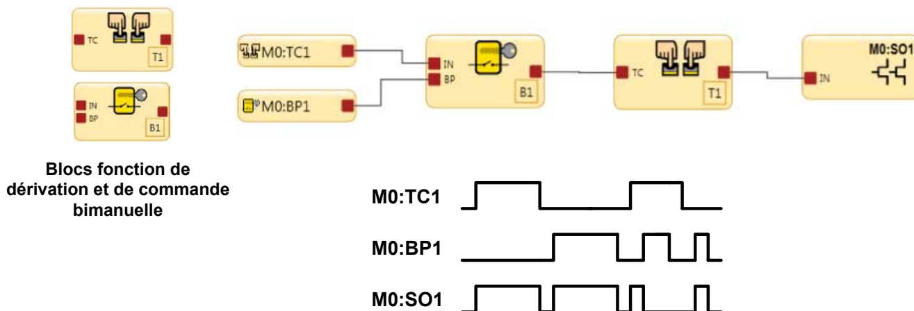
Illustration 143. Chronogramme — Bloc de commande bimanuelle et blocs de dérivation avec 1 entrée de commande bimanuelle
