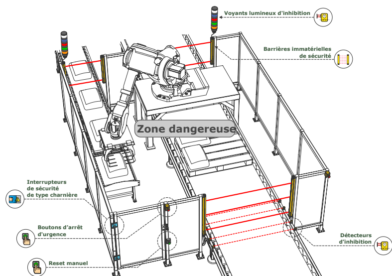
Illustration 13. Exemple d'installation - cellule robotisée
