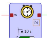
Illustration 105. Bloc de temporisation — Contrôleurs de base XS/SC26-2 FID 2 ou ultérieur et SC10-2
