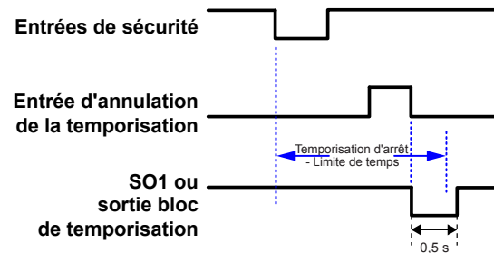
Illustration 21. Fonction Maintien de la sortie désactivée
