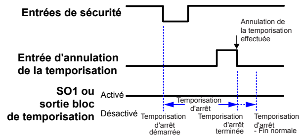
Illustration 30. Fonction Maintien de la sortie activée pour les entrées de sécurité sans reset de verrouillage
