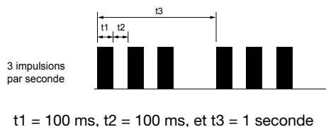
Illustration 47. 3 impulsions par seconde
