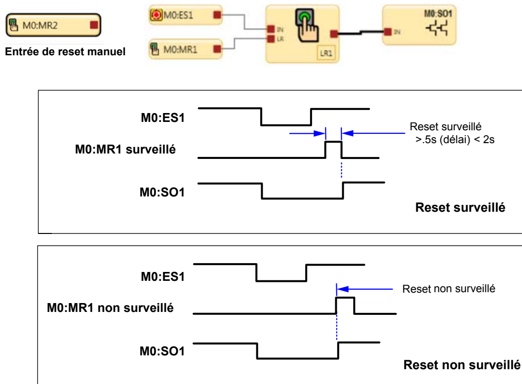
Illustration 114. Chronogramme — Bloc de reset à verrouillage, reset surveillé/non surveillé
