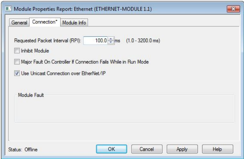
Illustration 178. Paramètres de connexion
