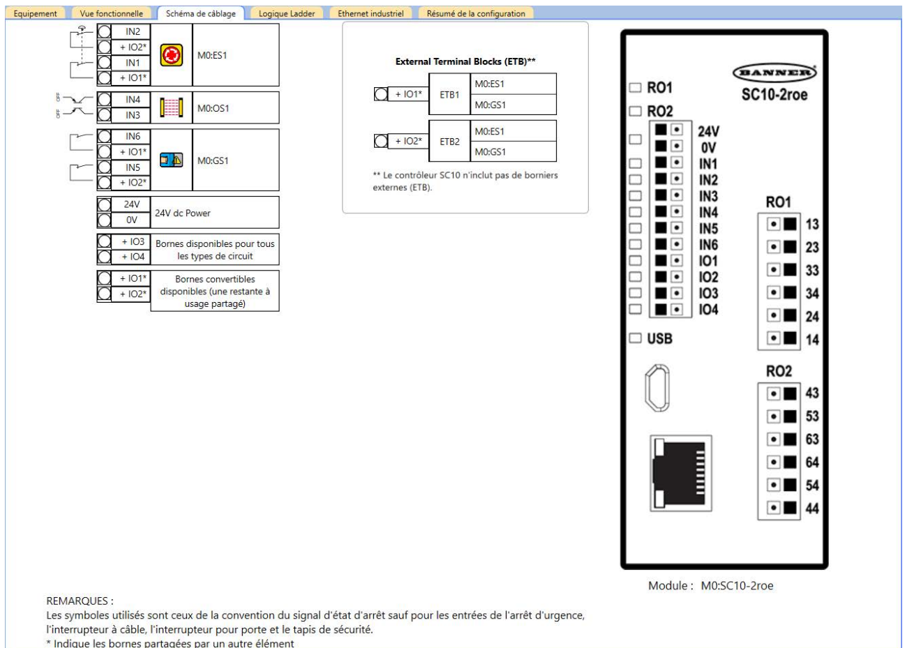
Illustration 251. Onglet Schéma de câblage avec bouton d'arrêt d'urgence, capteur optique, interrupteur de porte et borniers externes
