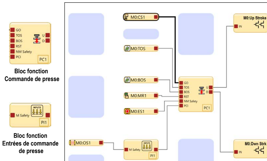
Illustration 136. Exemple de configuration pour une petite presse
