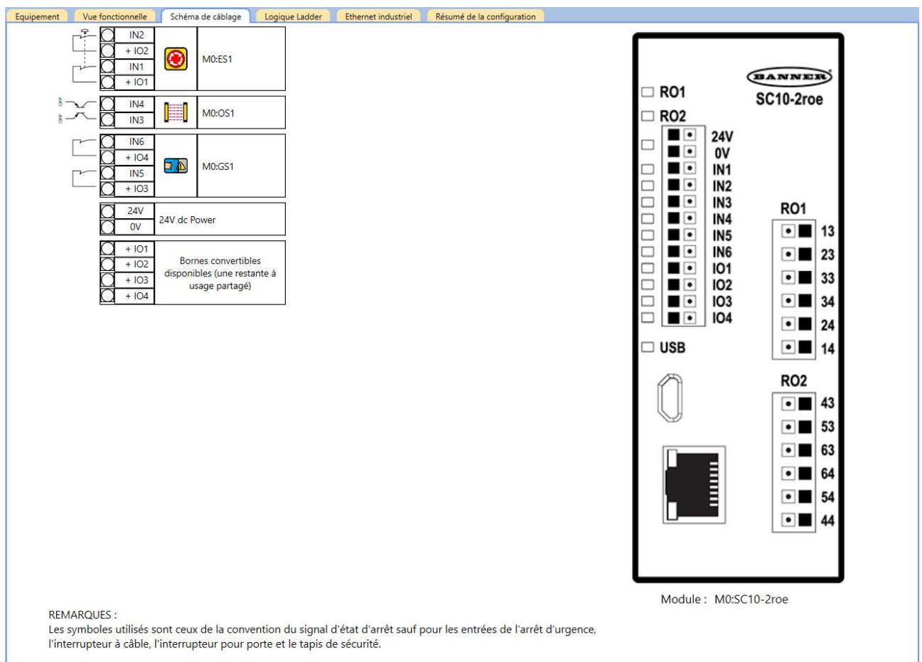
Illustration 249. Onglet Schéma de câblage avec bouton d'arrêt d'urgence, capteur optique et interrupteur de porte
