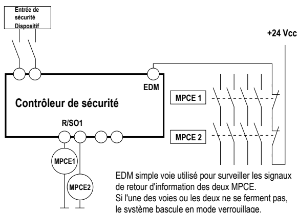
Illustration 37. Raccordement de l'EDM à un canal
