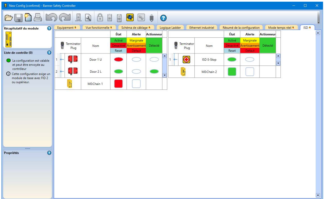
Illustration 80. Onglet ISD en mode temps réel avec un interrupteur ouvert
