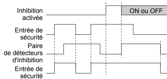
Illustration 127. Logique de temporisation — Paire de détecteurs d'inhibition avec inhibition activée
