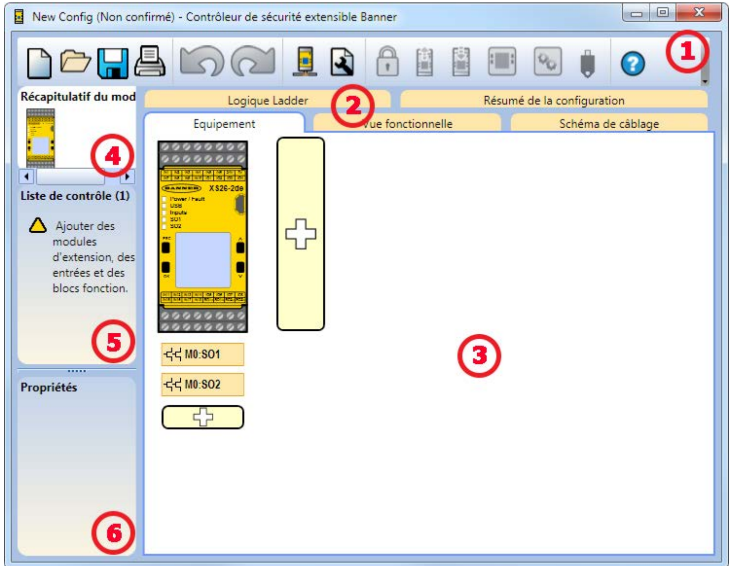
Illustration 67. Logiciel Contrôleur de sécurité Banner
