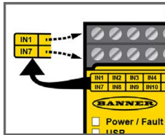
Illustration 15. Emplacement des bornes d'entrée et de sortie du XS/SC26-2
