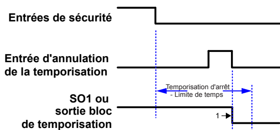
Illustration 27. L'entrée de sécurité reste en mode d'arrêt.
