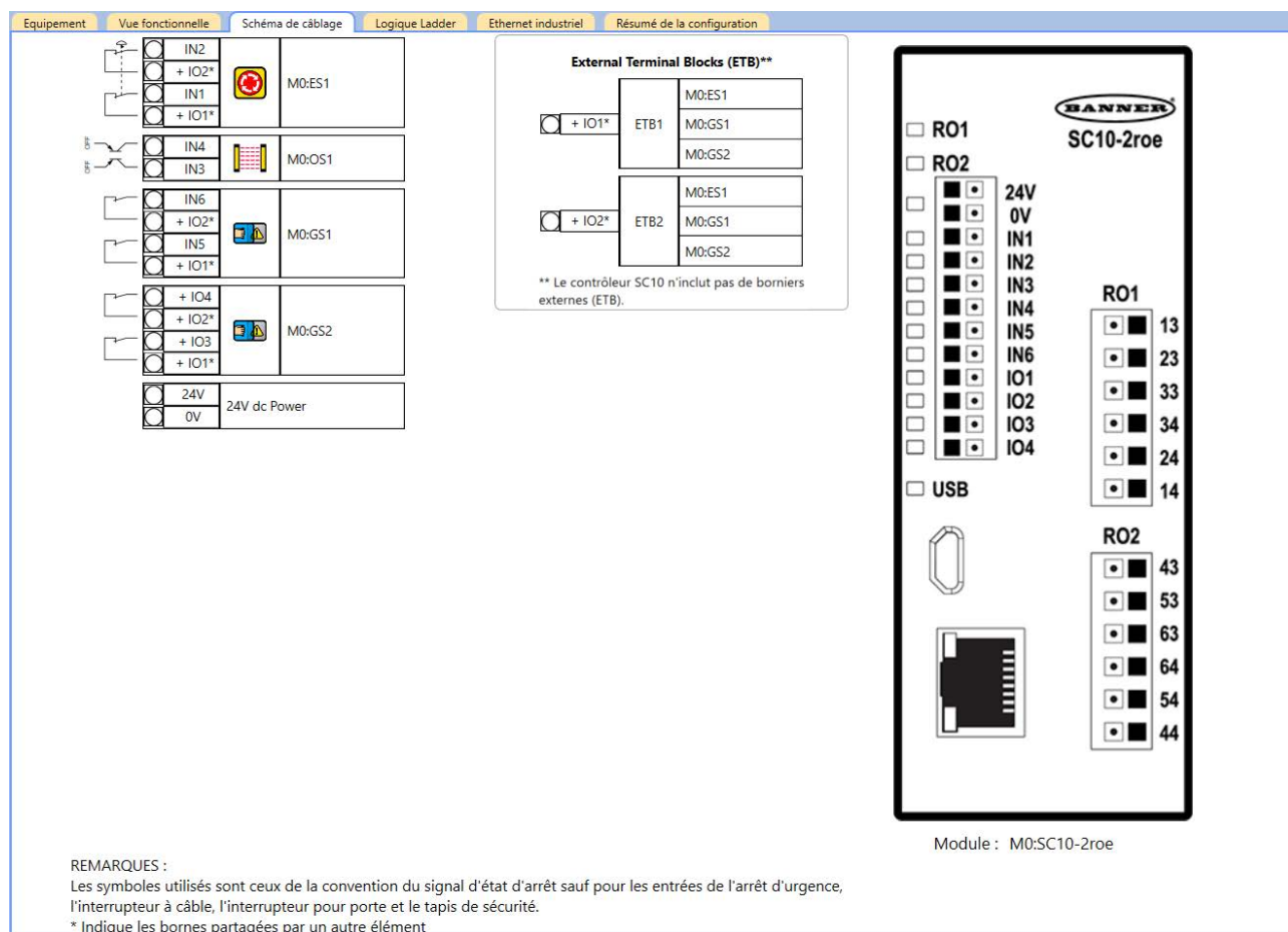
Illustration 252. Onglet Schéma de câblage avec bouton d'arrêt d'urgence, capteur optique, interrupteurs de porte et borniers externes
