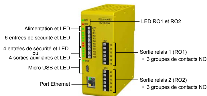
Illustration 7. Caractéristiques et indicateurs
