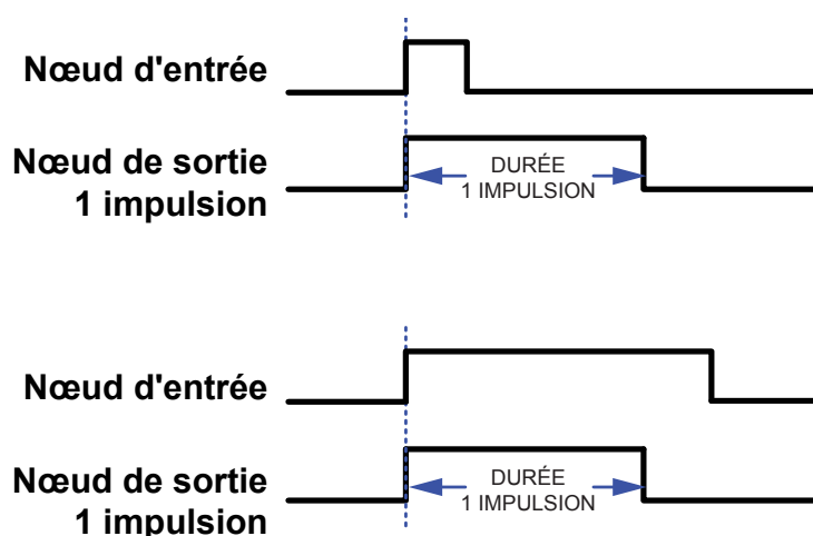
Illustration 129. Diagrammes de synchronisation 1 impulsion en mode normal
