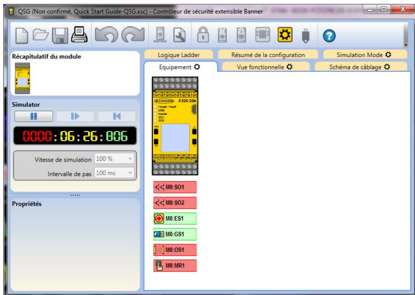
Illustration 99. Mode simulation — Onglet Équipement
