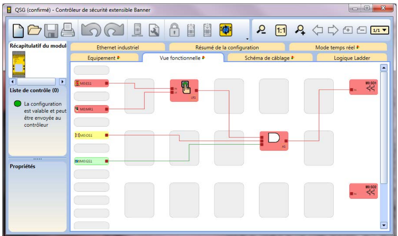
Illustration 95. Temps d'exécution — Onglet Vue fonctionnelle
