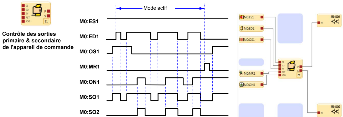
Illustration 112. Chronogramme — Appareil (dispositif) de commande
