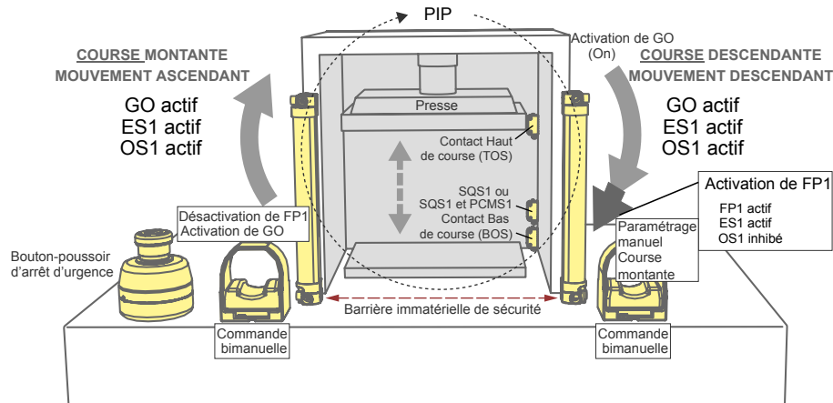
Illustration 63. Configuration d'une commande de presse avec fonctionnalités complètes
