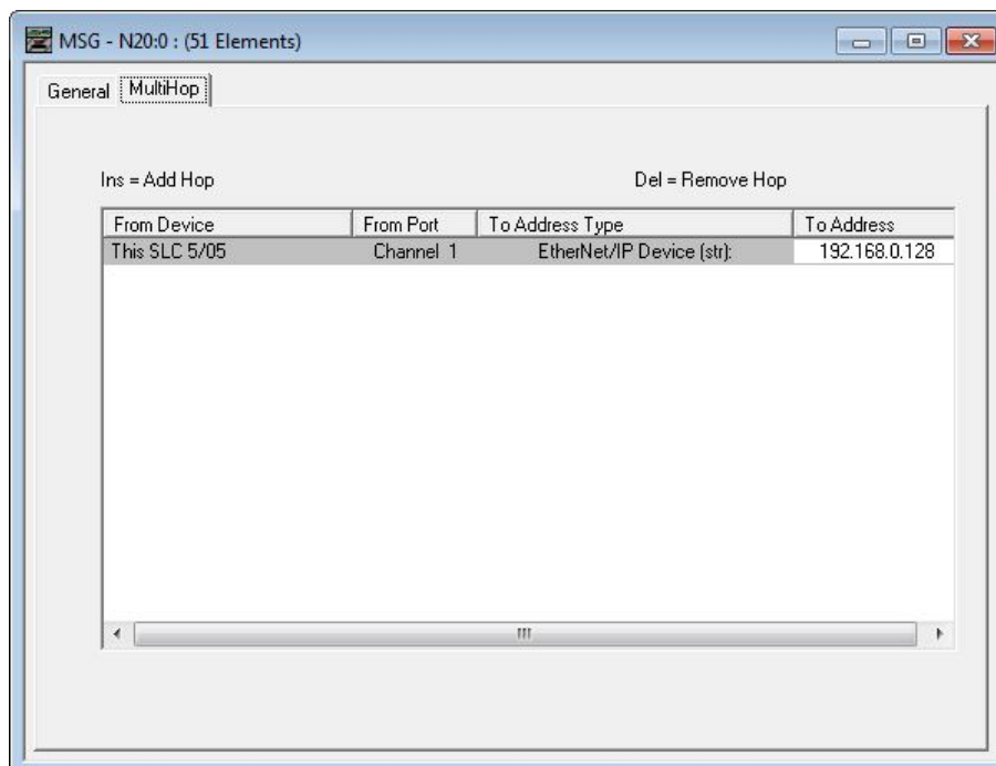
Illustration 226. Fenêtre MSG - N20:0 (51 éléments) — Onglet Multi-sauts
