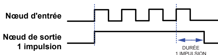
Illustration 130. Diagramme de synchronisation 1 impulsion en mode pulsation
