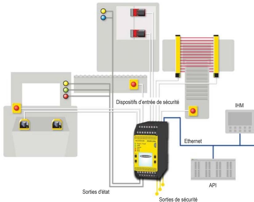
Illustration 3. Sorties de sécurité (exemple d'application)
