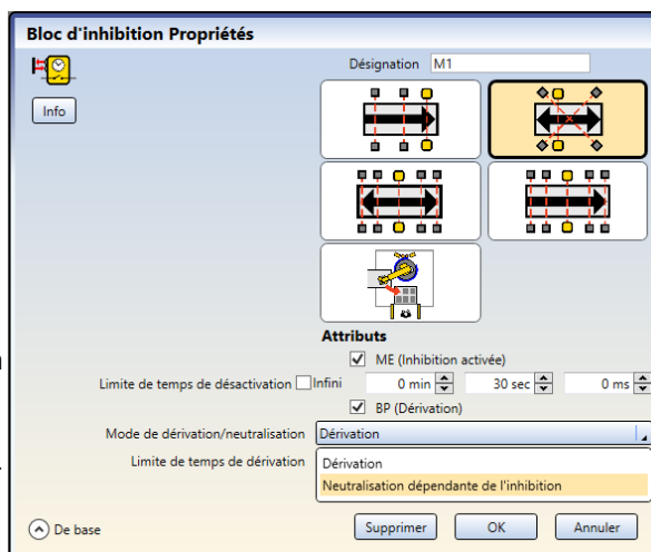
Illustration 120. Neutralisation dépendante de l'inhibition
