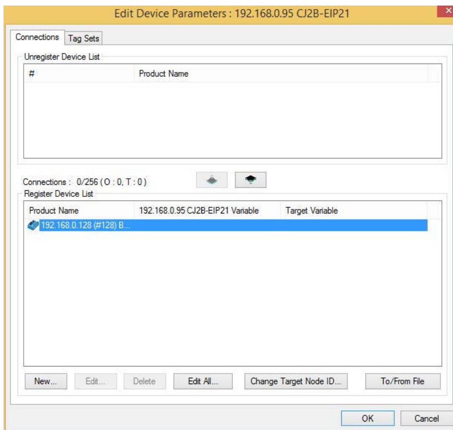
Illustration 203. Register Device List (Liste des dispositifs enregistrés)
