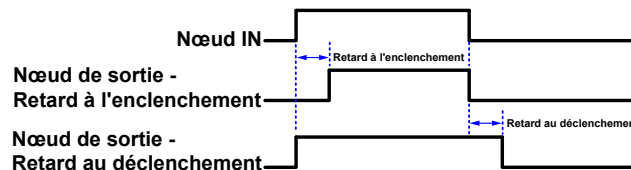
Illustration 109. Schéma de temps d'un bloc de temporisation
