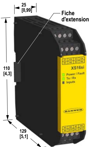
Illustration 11. Dimensions du module d'extension
