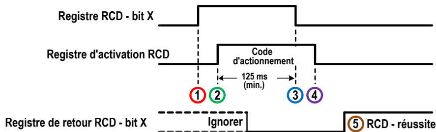
Illustration 26. Séquence de reset ou d'annulation de la temporisation — Méthode avec délai
