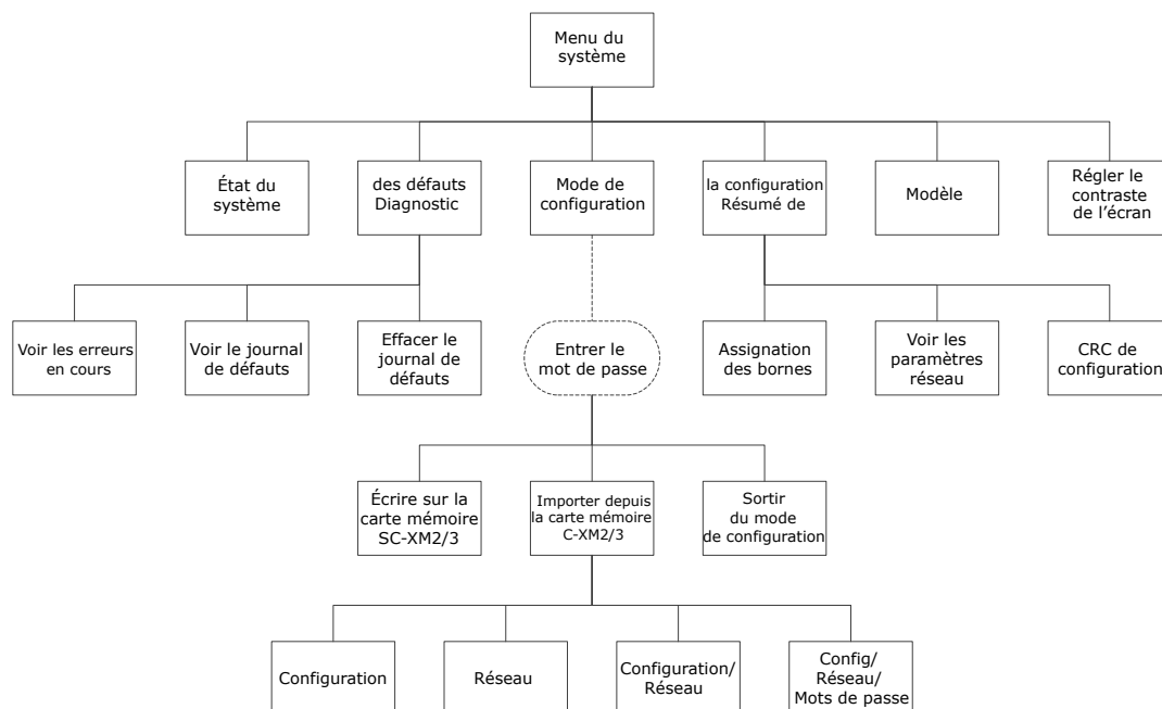
Illustration 147. Carte de l'interface embarquée
