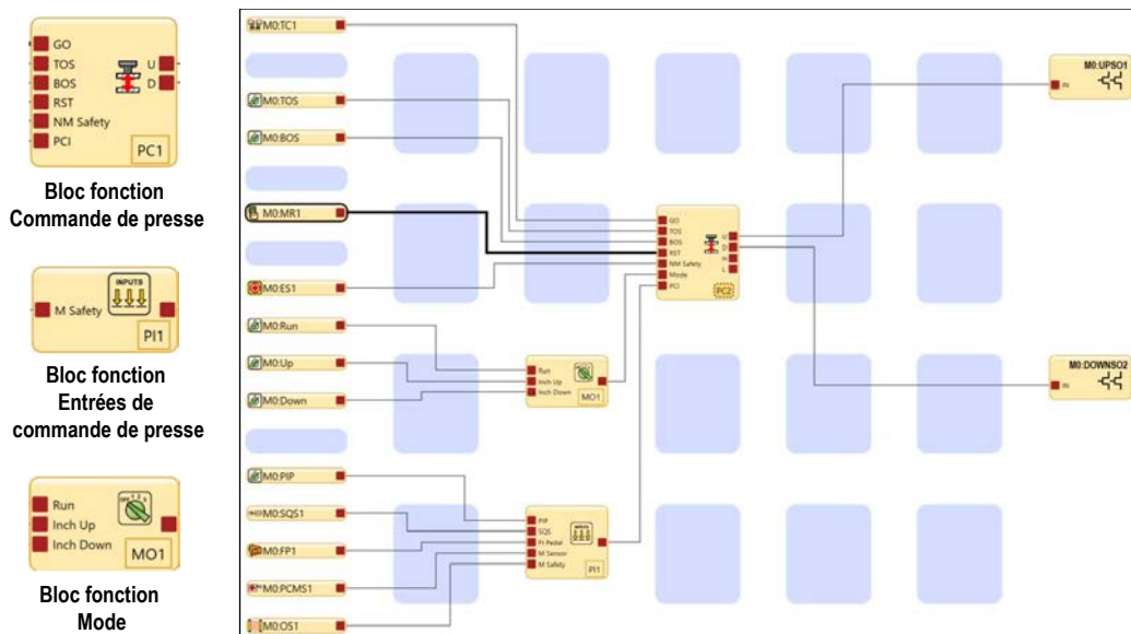
Illustration 138. Commande de presse — Exemple de configuration
