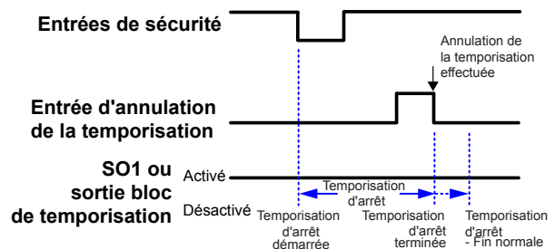
Illustration 23. Fonction Maintien de la sortie activée pour les entrées de sécurité sans reset de verrouillage
