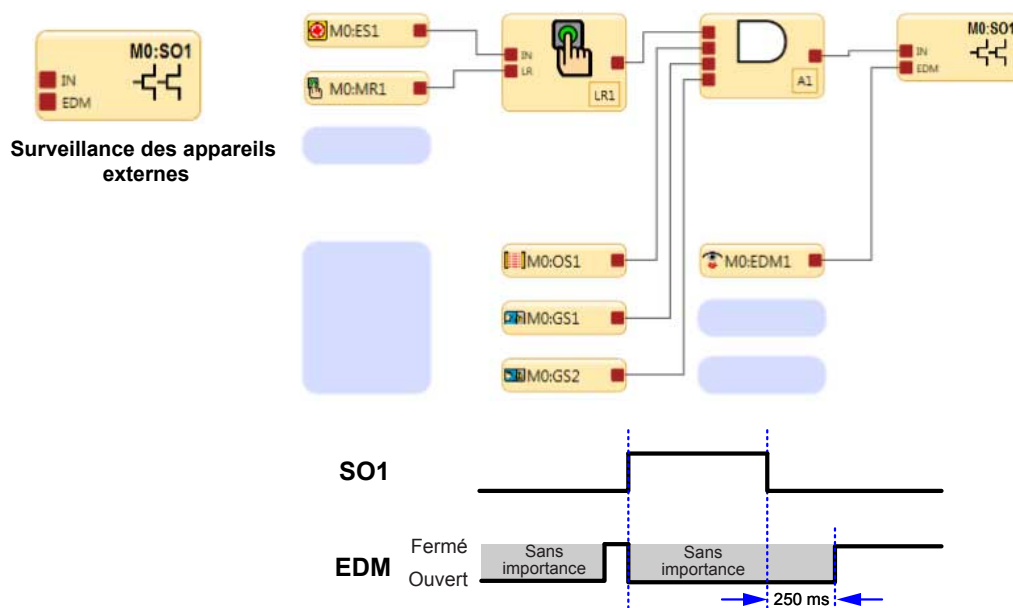
Illustration 39. Logique de temporisation : Etat de l'EDM à un canal par rapport à la sortie de sécurité
