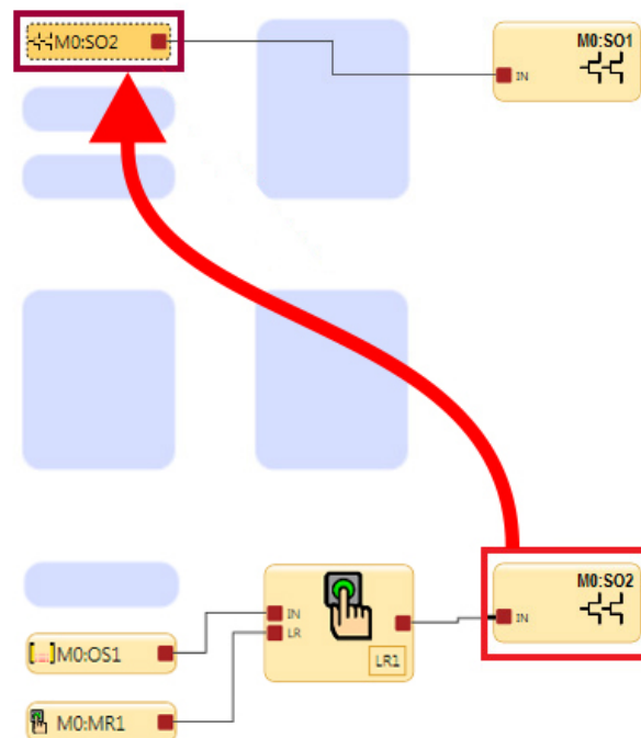
Illustration 107. Sortie de sécurité contrôlée par une autre sortie de sécurité
