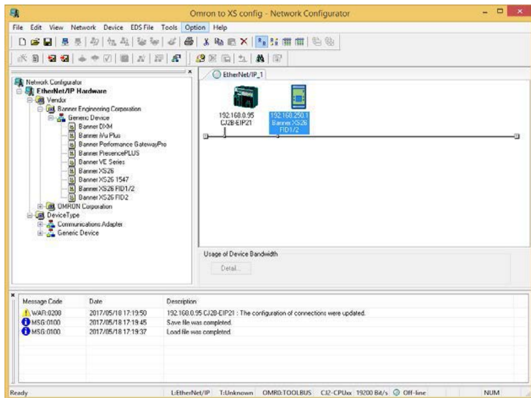
Illustration 200. Ajout du contrôleur de sécurité
