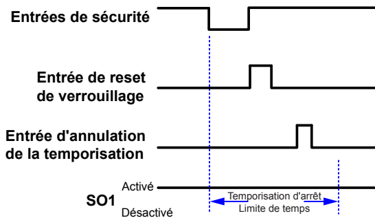
Illustration 22. Fonction Maintien de la sortie activée pour les entrées de sécurité avec reset de verrouillage
