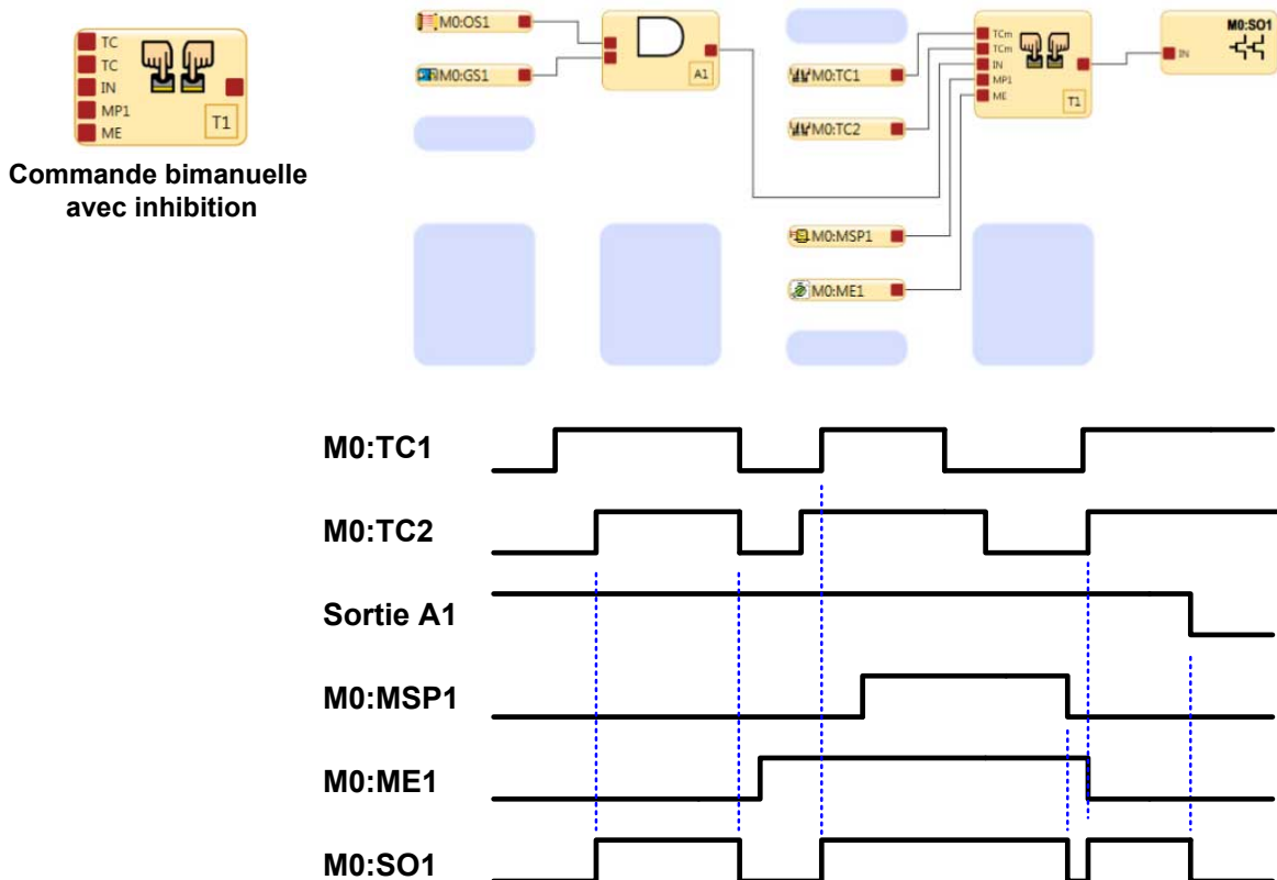
Illustration 146. Chronogramme — Bloc de commande bimanuelle avec inhibition
