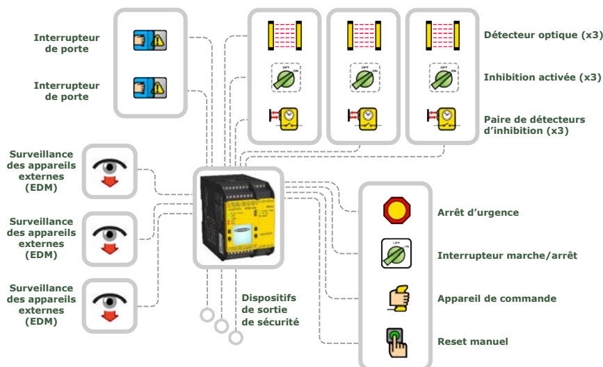
Illustration 57. Schéma de l'exemple de configuration
