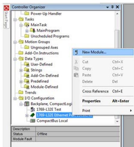
Illustration 166. Ajout d'un module Ethernet
