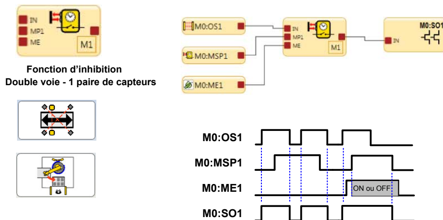
Illustration 124. Chronogramme — Bloc d'inhibition double canal, une paire de détecteurs d'inhibition
