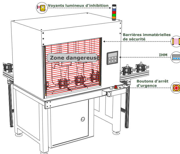
Illustration 14. Exemple d'application du SC10-2
