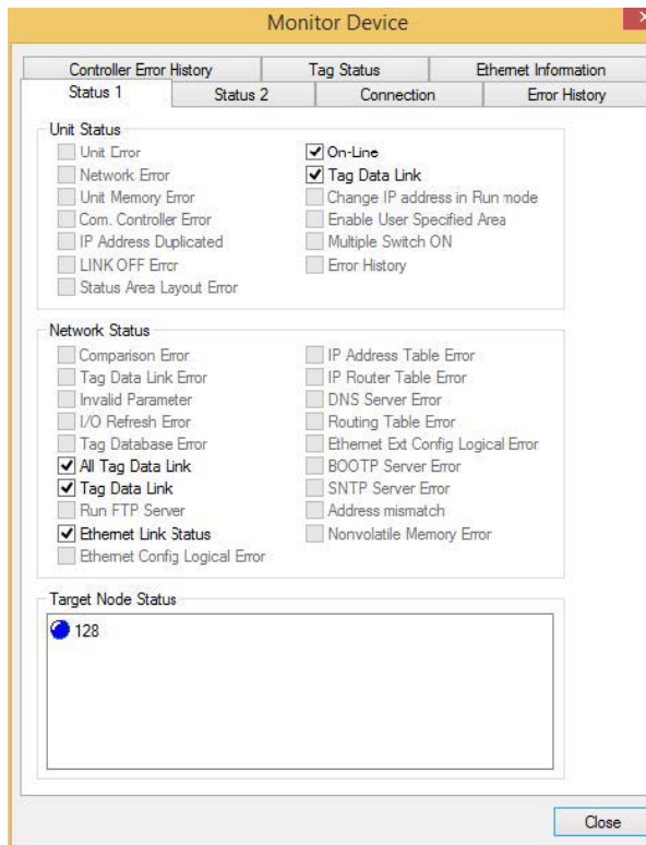
Illustration 216. Fenêtre Monitor Device — Onglet Status 1
