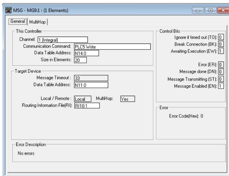
Illustration 227. Fenêtre MSG - MG9:1 (1 élément) — Onglet Général
