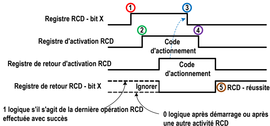
Illustration 25. Séquence de reset ou d'annulation de la temporisation — Méthode avec retour
