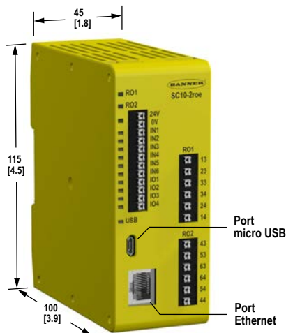
Illustration 12. Dimensions du SC10-2
