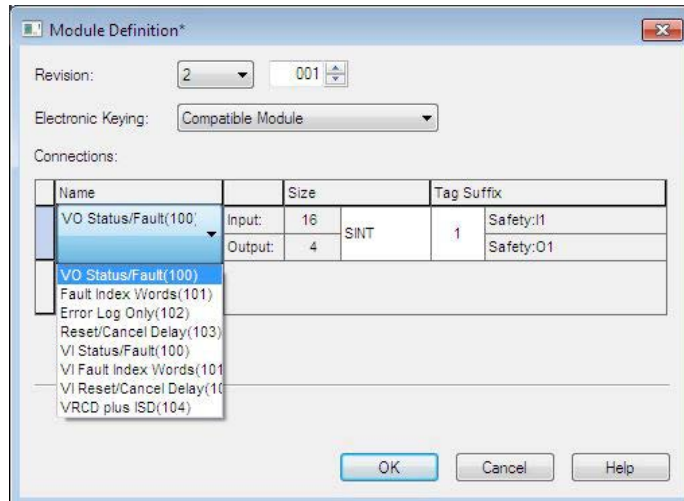
Illustration 160. Définition du module
