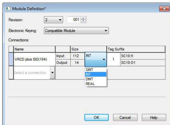
Illustration 161. Définition du module — Type de données
