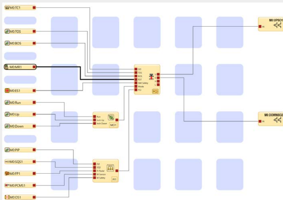
Illustration 66. Position des blocs fonction
