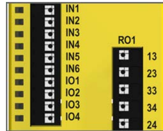
Illustration 16. Emplacement des bornes d'entrée et de sortie du SC10-2
