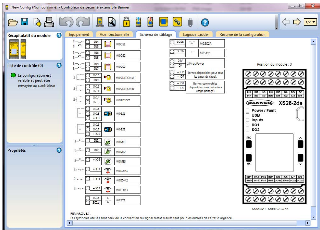
Illustration 76. Onglet Schéma de câblage — XS26-2
