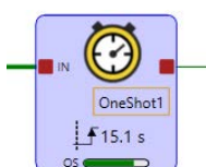
Illustration 106. Bloc de temporisation — Contrôleurs de base XS/SC26-2 FID 4 ou ultérieur uniquement
