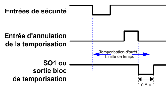
Illustration 28. Fonction Maintien de la sortie désactivée
