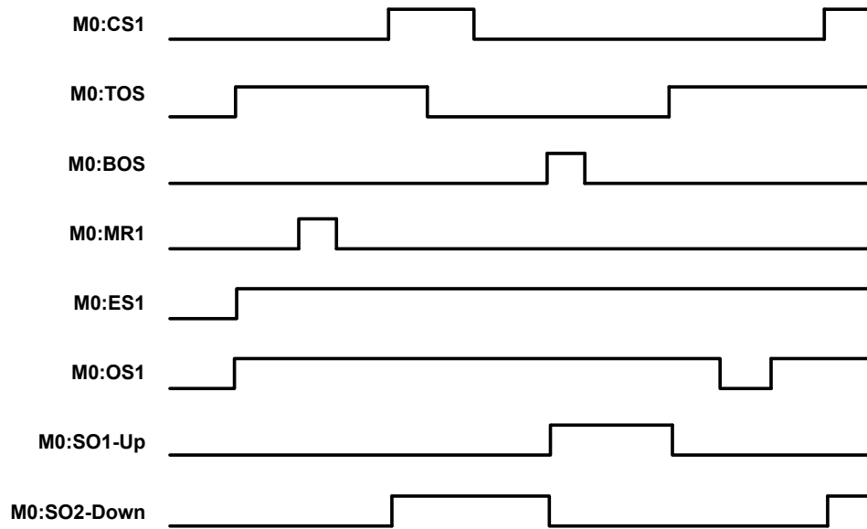
Illustration 137. Commande de la presse — Diagramme temporel, commande à actionneur unique
