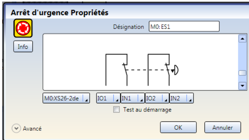
Illustration 52. Paramètres d'entrée de sécurité de base
