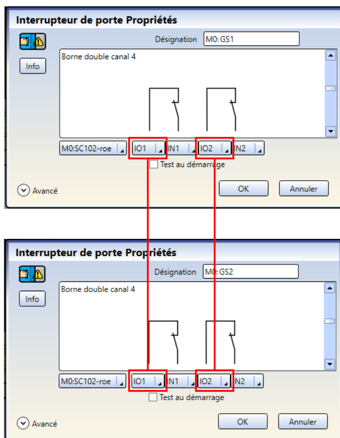
Illustration 4. Partage de IO1 et IO2 par GS1 et GS2
