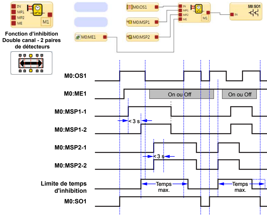
Illustration 126. Arrêt d'urgence et fonction d'inhibition
