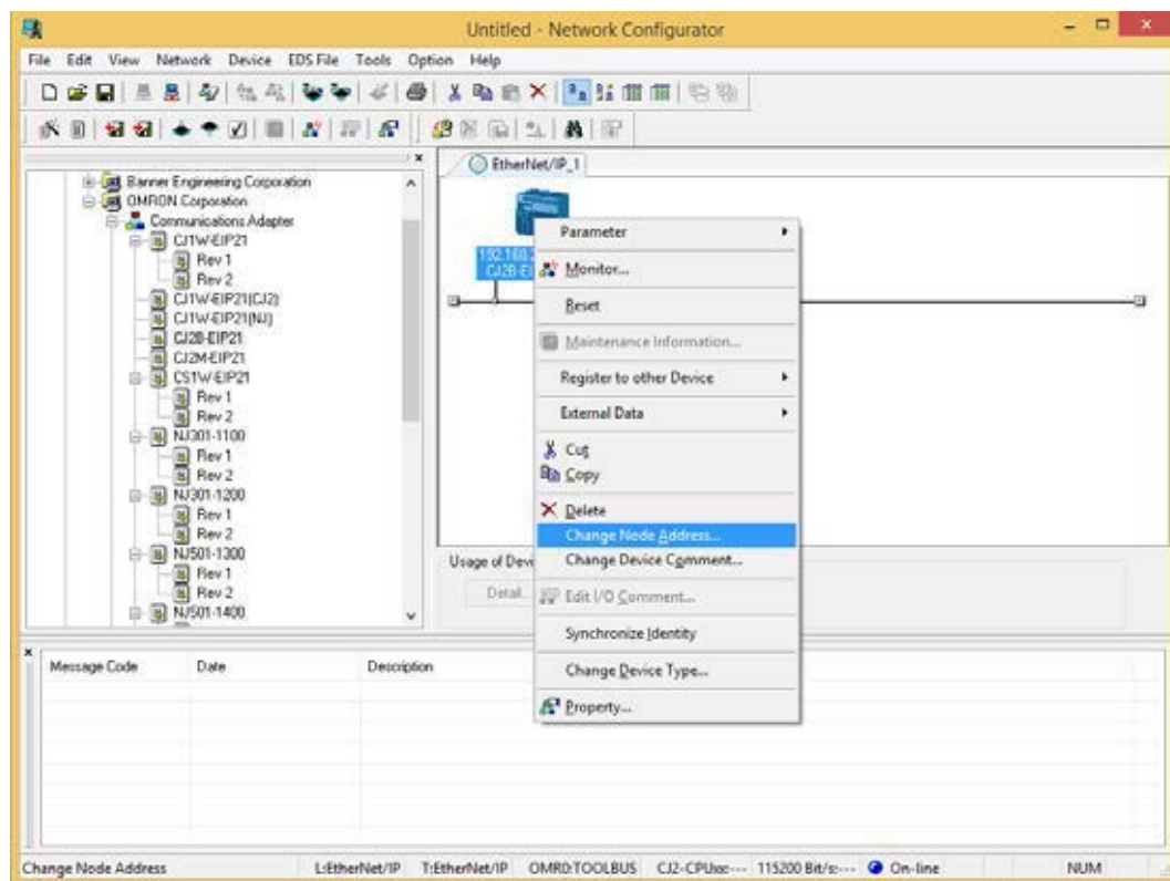
Illustration 198. Menu contextuel
