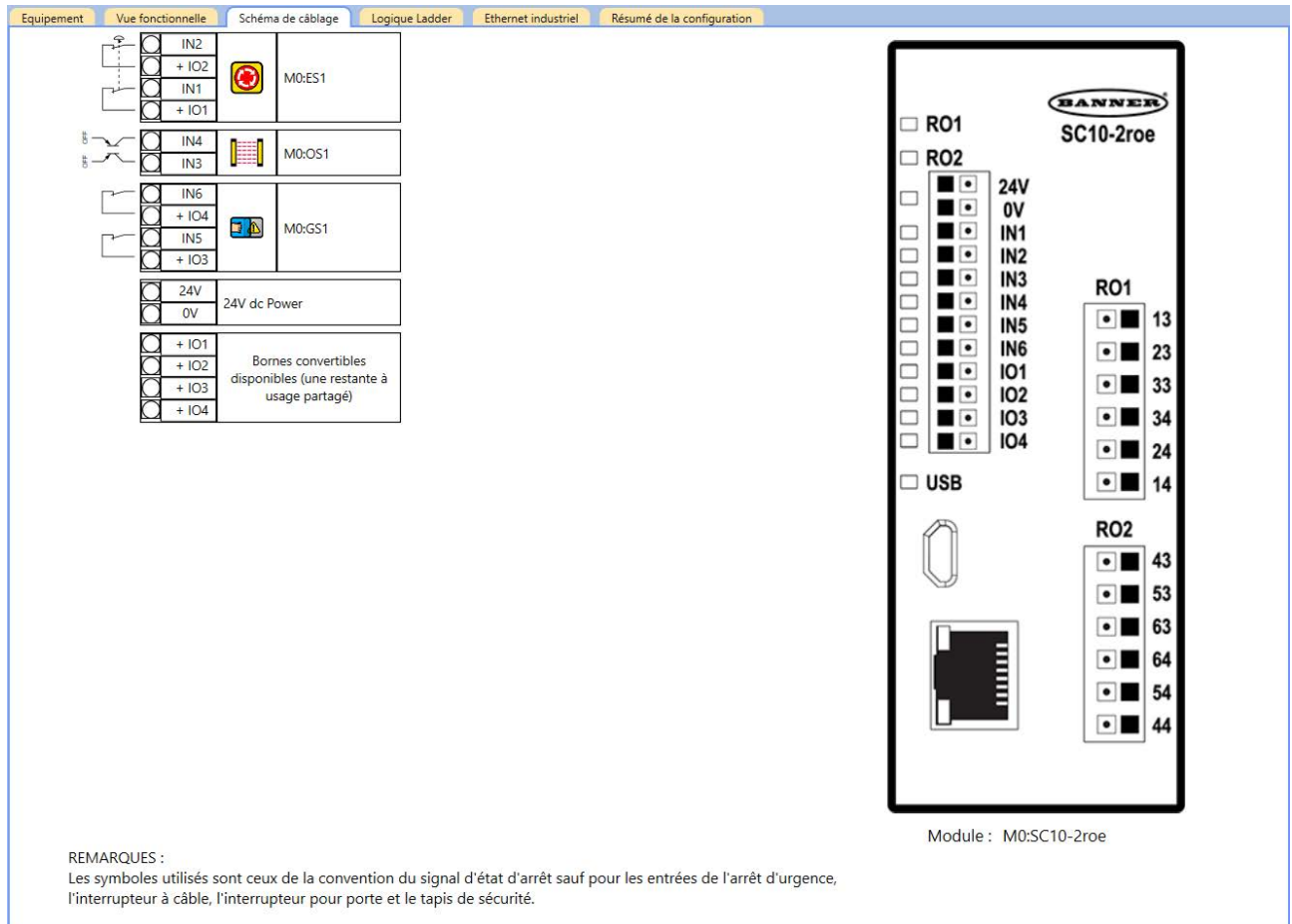
Illustration 246. Onglet Schéma de câblage avec bouton d'arrêt d'urgence, capteur optique et interrupteur de porte
