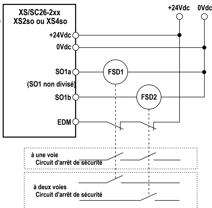
Illustration 42. Raccordement générique du XS/SC26-2 : sortie de sécurité électronique avec EDM
