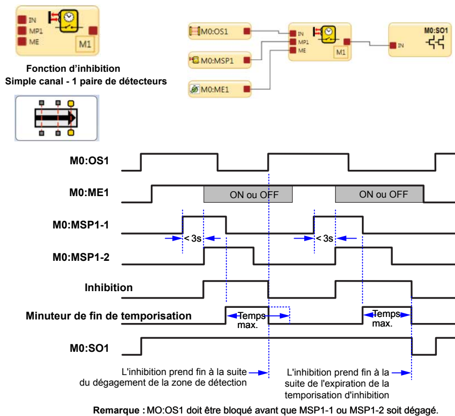
Illustration 122. Chronogramme — Bloc d'inhibition simple canal, une paire de détecteurs d'inhibition
