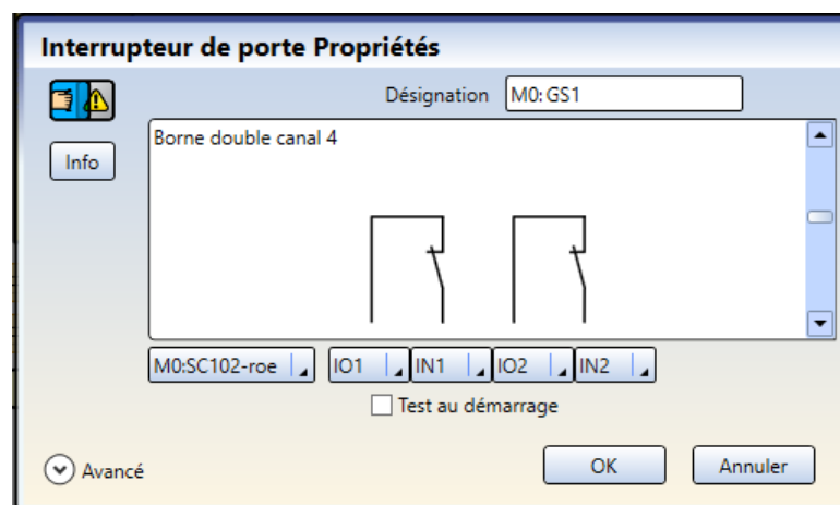
Illustration 250. Propriétés de l'interrupteur de porte
