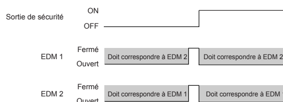
Illustration 41. Logique de temporisation : Etat de l'EDM à deux canaux par rapport à la sortie de sécurité
