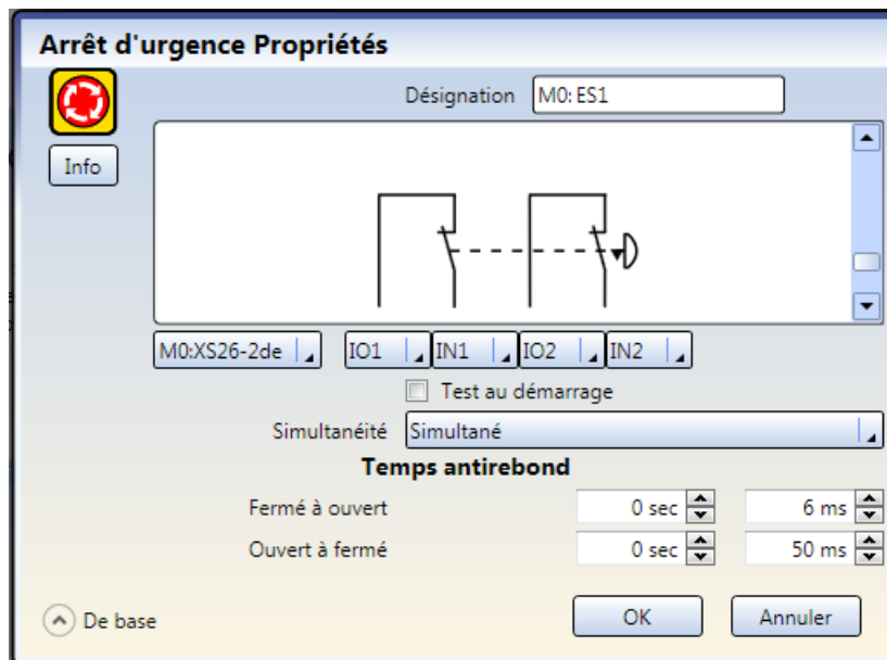
Illustration 53. Paramètres d'entrée de sécurité avancés
