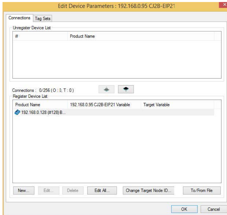
Illustration 211. Fenêtre Edit Device Parameters — Onglet Connections
