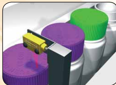
Application typique en suppression d'arrière-plan fixe : présence de bouchon
