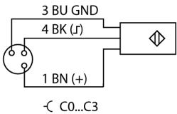
Ausgang M8 x 1
