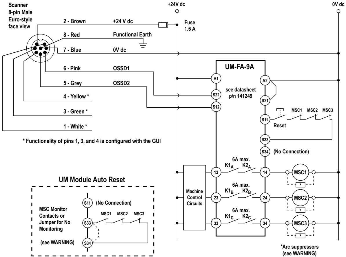
Figure 38. Wiring using a UM module
