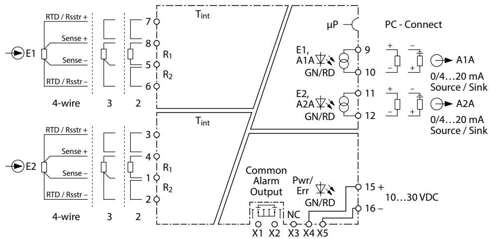
Abb. 7: IM12-TI01-2RTDR-2I
