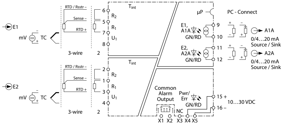
Abb. 9: IM12-TI02-2TCURTDR-2I
